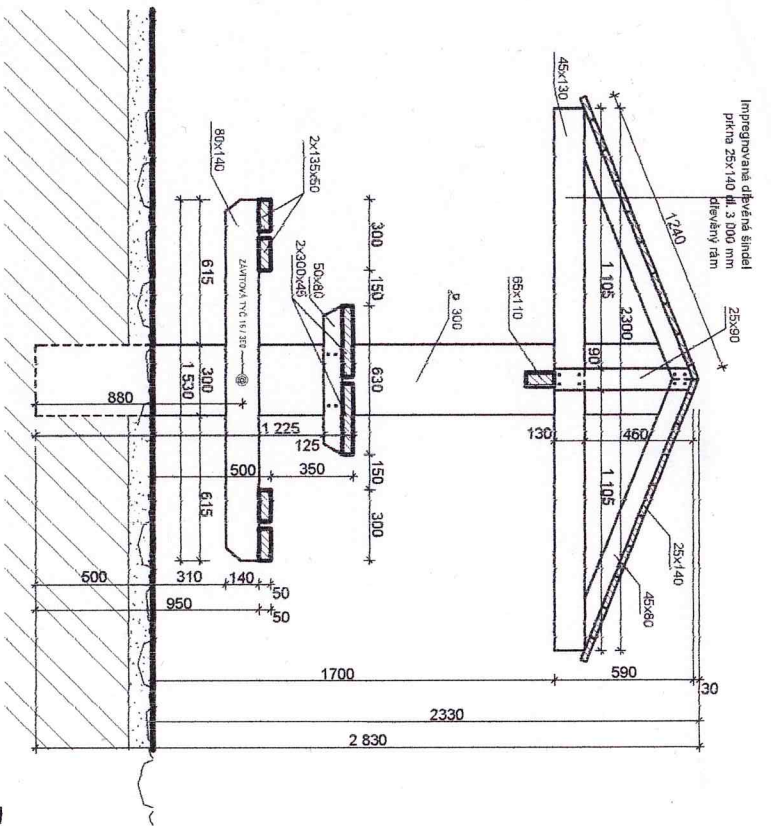
Řez příčný
